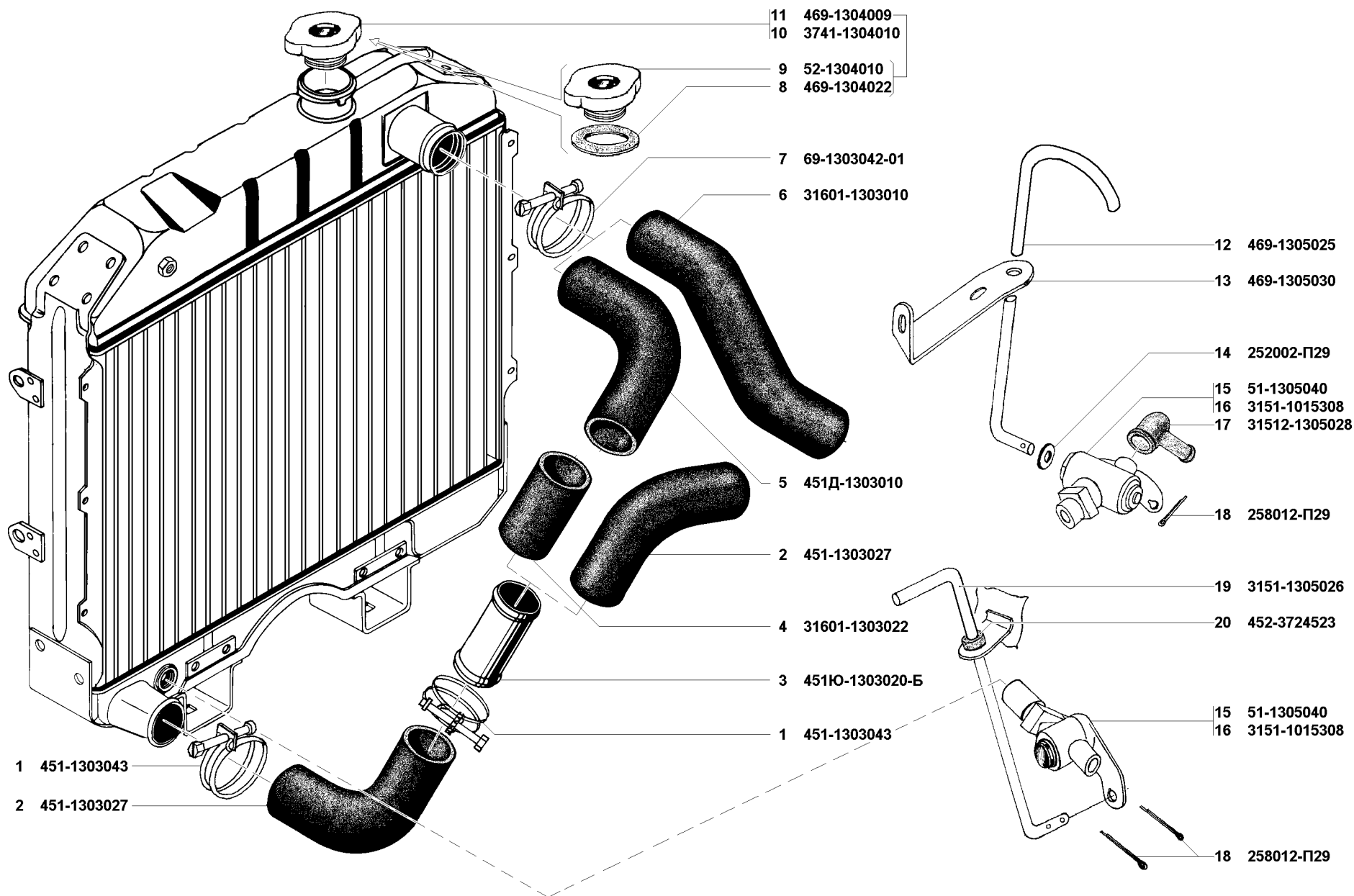
Рис. 33. Трубопроводы и шланги (1303), пробка радиатора (1304) и краник сливной (1305)
